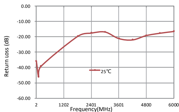
RF端回波损耗
