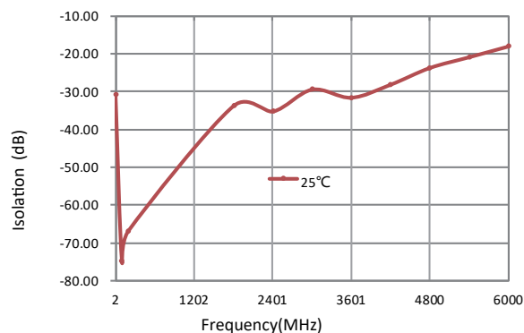
RF-DC隔离度
