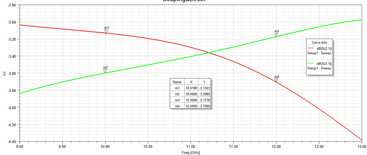
Amplitude_balance
