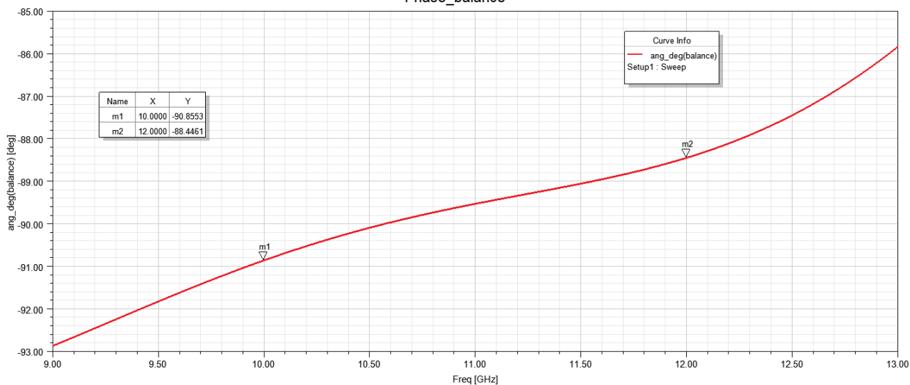
Phase_balance
